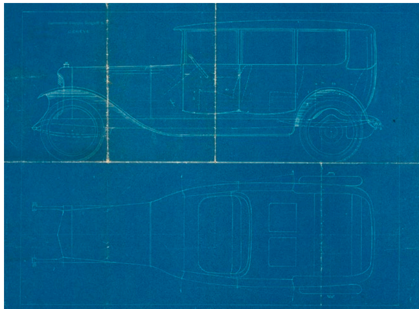
Plan bleu de la Delaunay-Belleville de Robert Hofmann (probablement années 1920). Fonds partiellement traité en 2020.
